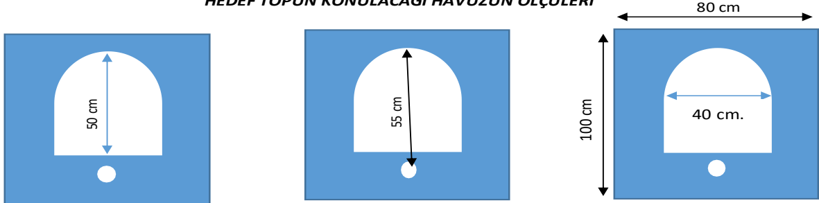
HEDEF TOPUN KONULACAĞI HAVUZUN ÖLÇÜLERİ
